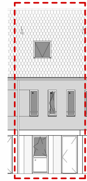
voorgevel (W)
